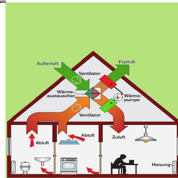
funktionsschema luftwärmepumpe
