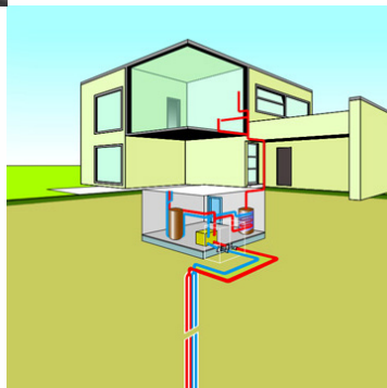
funktionsschema erdsondewärmepumpe
